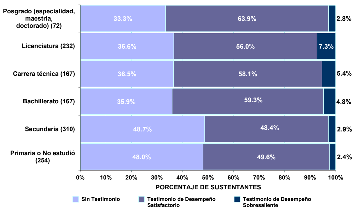
Gráfica 28. Distribución de la población en testimonios de desempeño por escolaridad de la madre .
