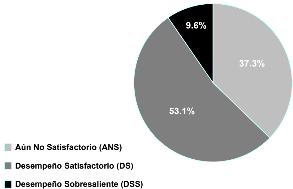
Gráfica 14. Distribución en niveles de desempeño del conjunto de sustentantes del EGEL durante 2017. Área Investigación
