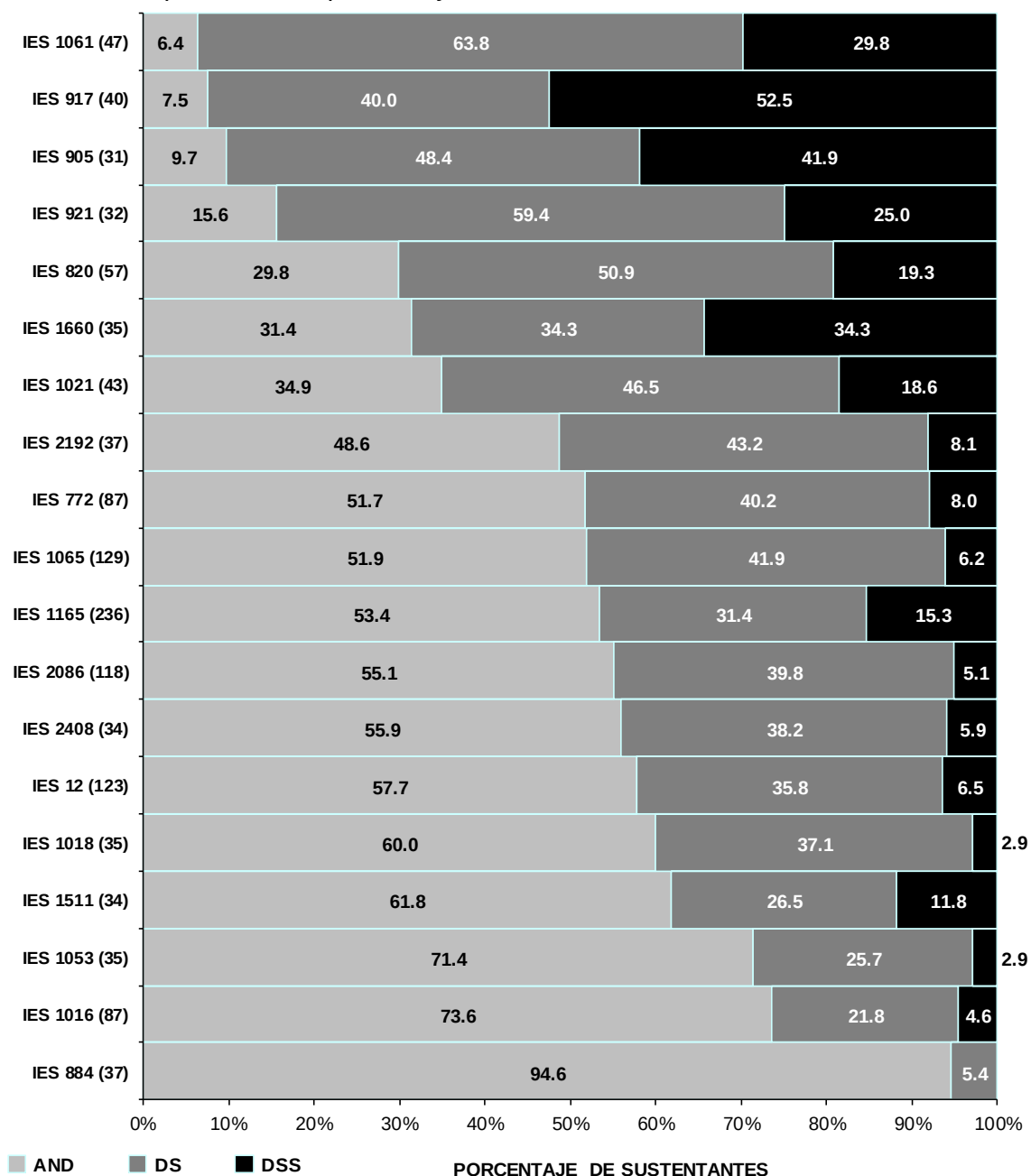
Gráfica 18. Distribución en niveles de desempeño por institución de procedencia (IES con 30 o más sustentantes) en el área Operación y mantenimiento de sistemas electrónicos
