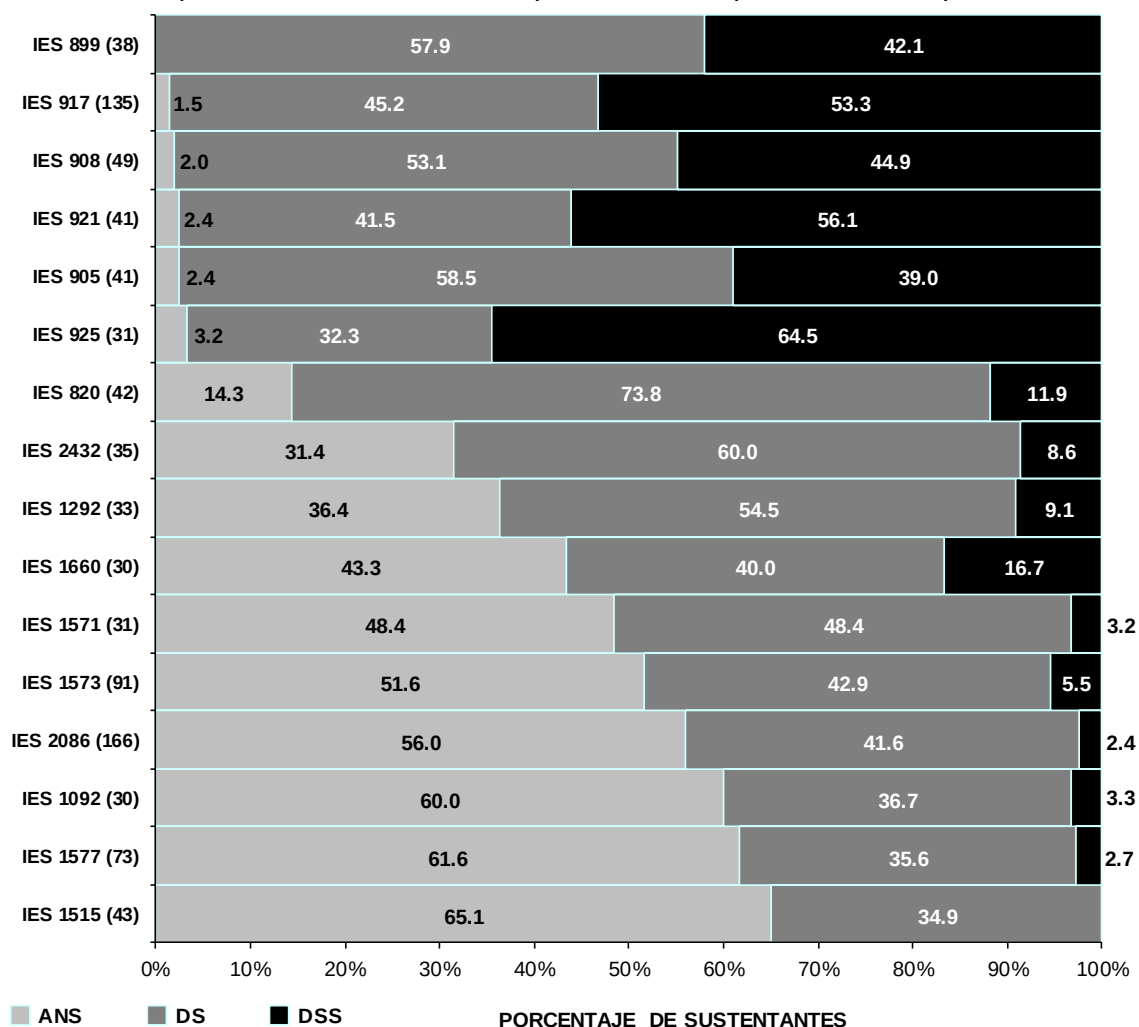
Gráfica 14. Distribución en niveles de desempeño por institución de procedencia (IES con 30 o más sustentantes) en el área Desarrollo e implantación de aplicaciones computacionales
